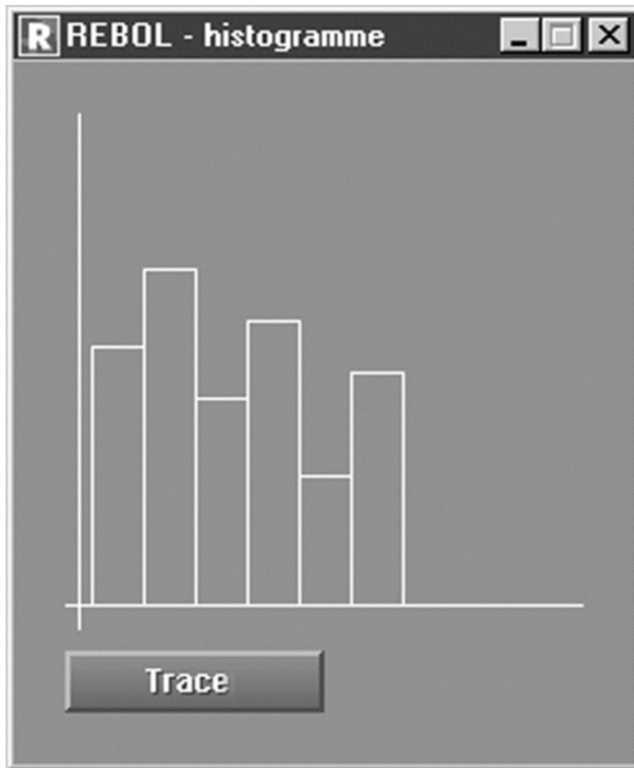
Рисунок 3-10. Сгенерированная гистограмма
