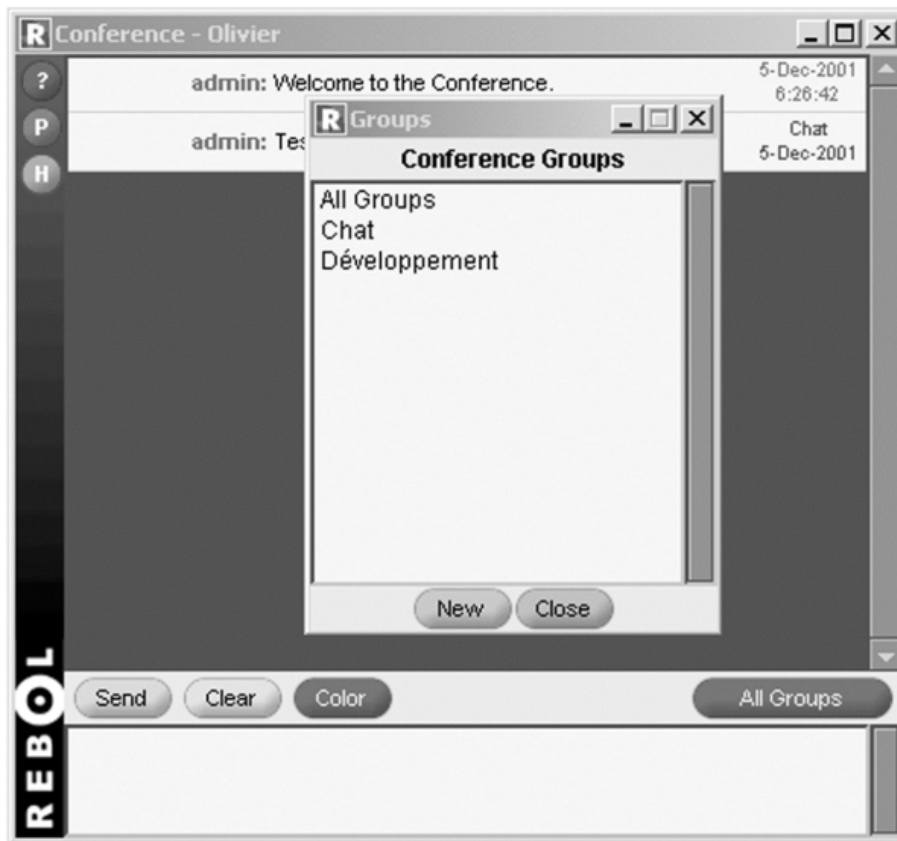
Рисунок 5-8. Конференция реблетка.
