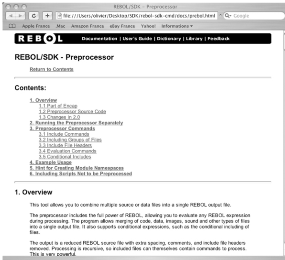
Рисунок 5-13. Документация препроцессора.
