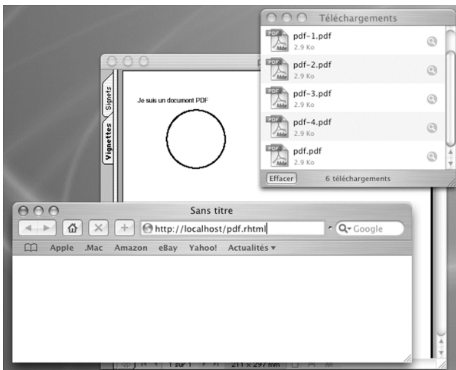
Рисунок 4-10. Создание PDF-документов.
