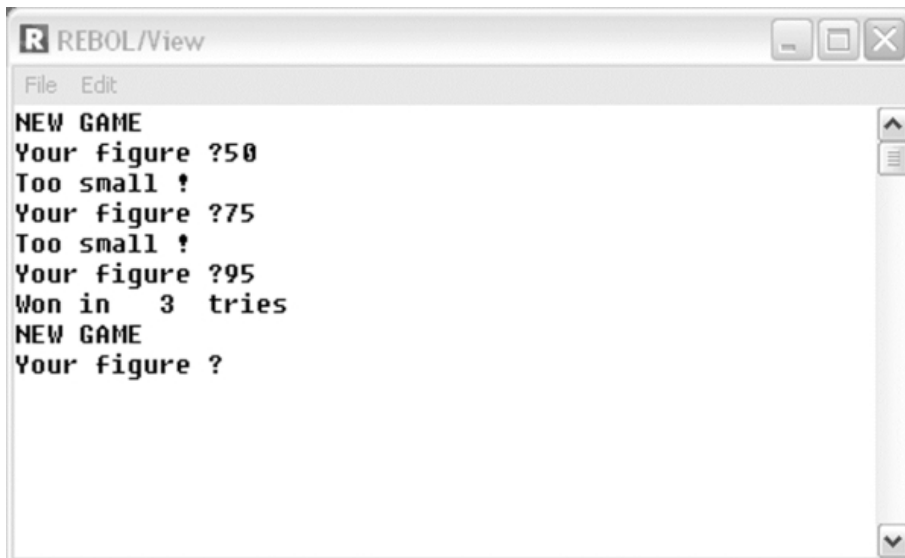
Рисунок 2-2. Запускаем игру.
