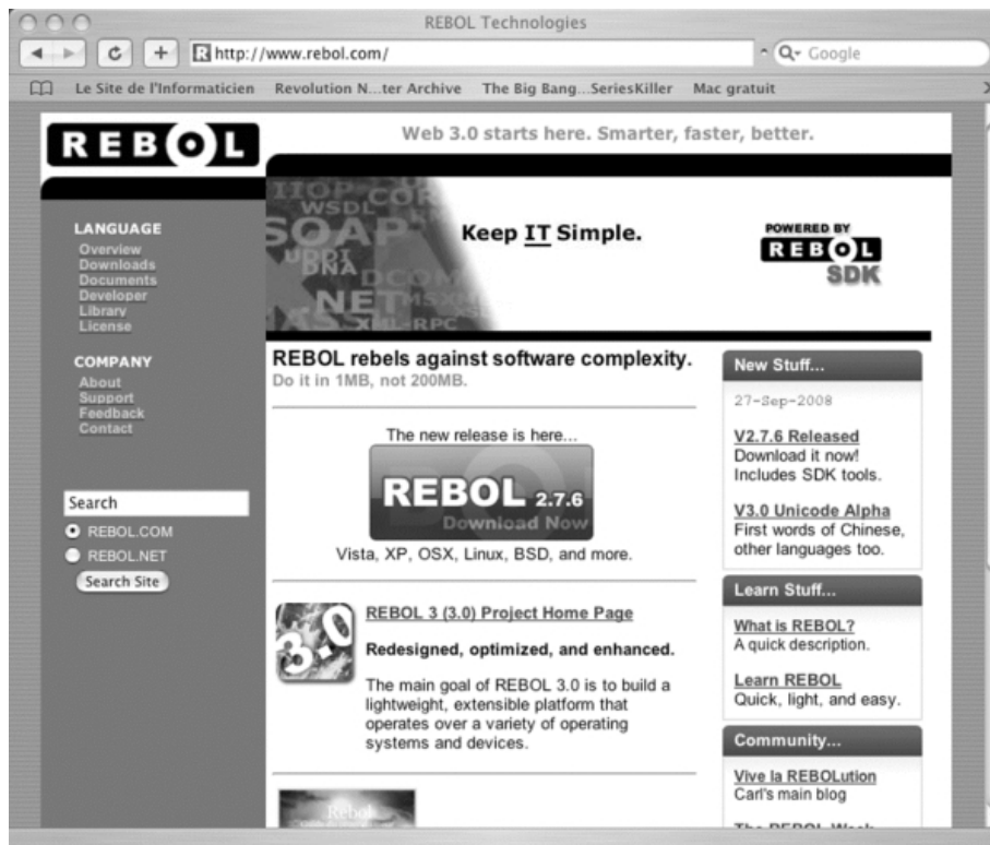
Рисунок 0-8. Сайт www.rebol.com.
