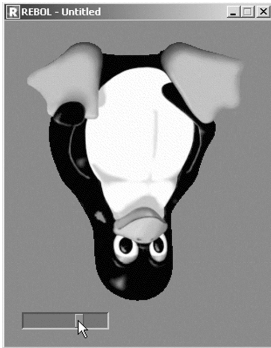
Рисунок 3-5. Поворот изображения
