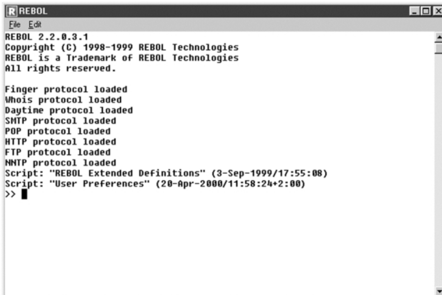
Рисунок 0-2. Консоль Rebol/Core.
